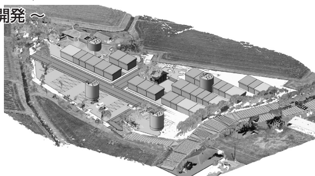
仮設住宅の配置案自動作成結果の一例。点群から自動作成した敷地の3Dモデルに住戸のボリュウムモデルが自動で配置される。
