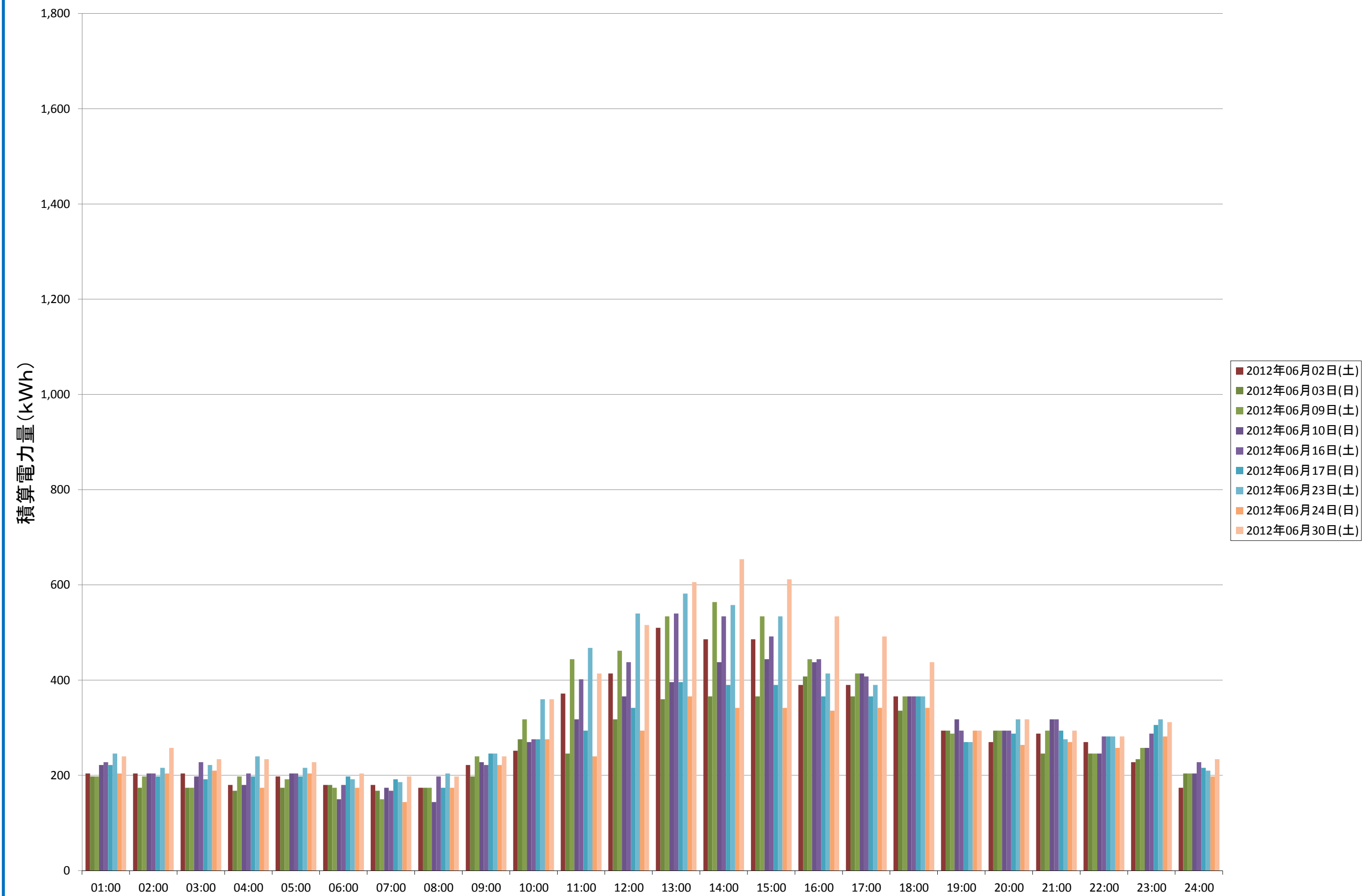
黒髪北キャンパス 6月の使用電力量(土日祝)
