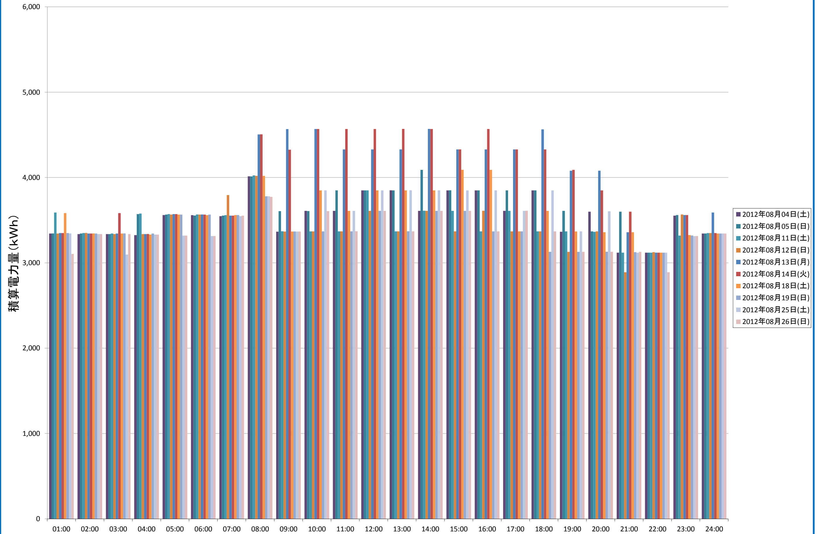
本荘北キャンパス 8月の使用電力量(土日祝)
