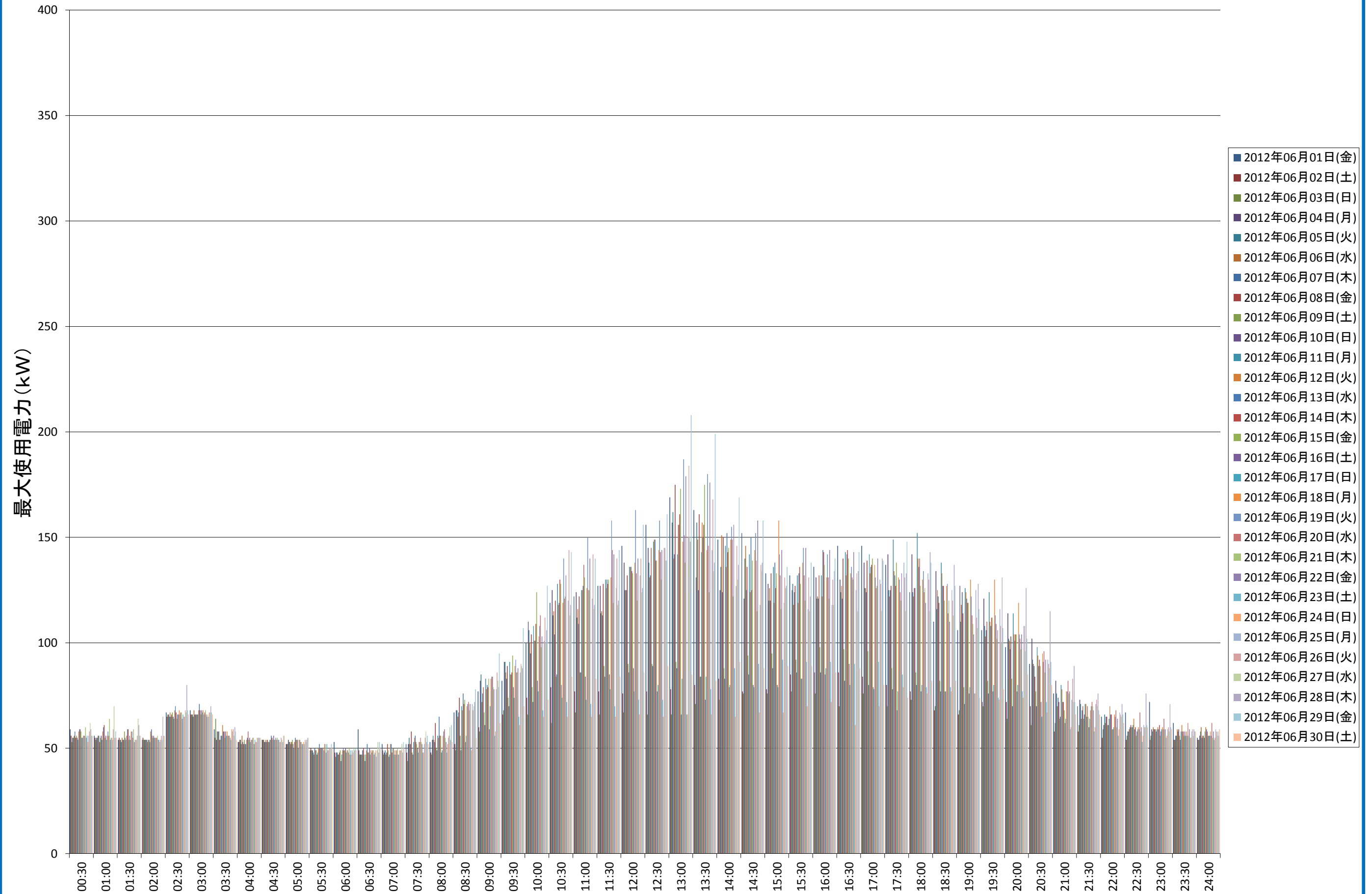
本荘南キャンパス 6月の時間帯別最大使用電力
