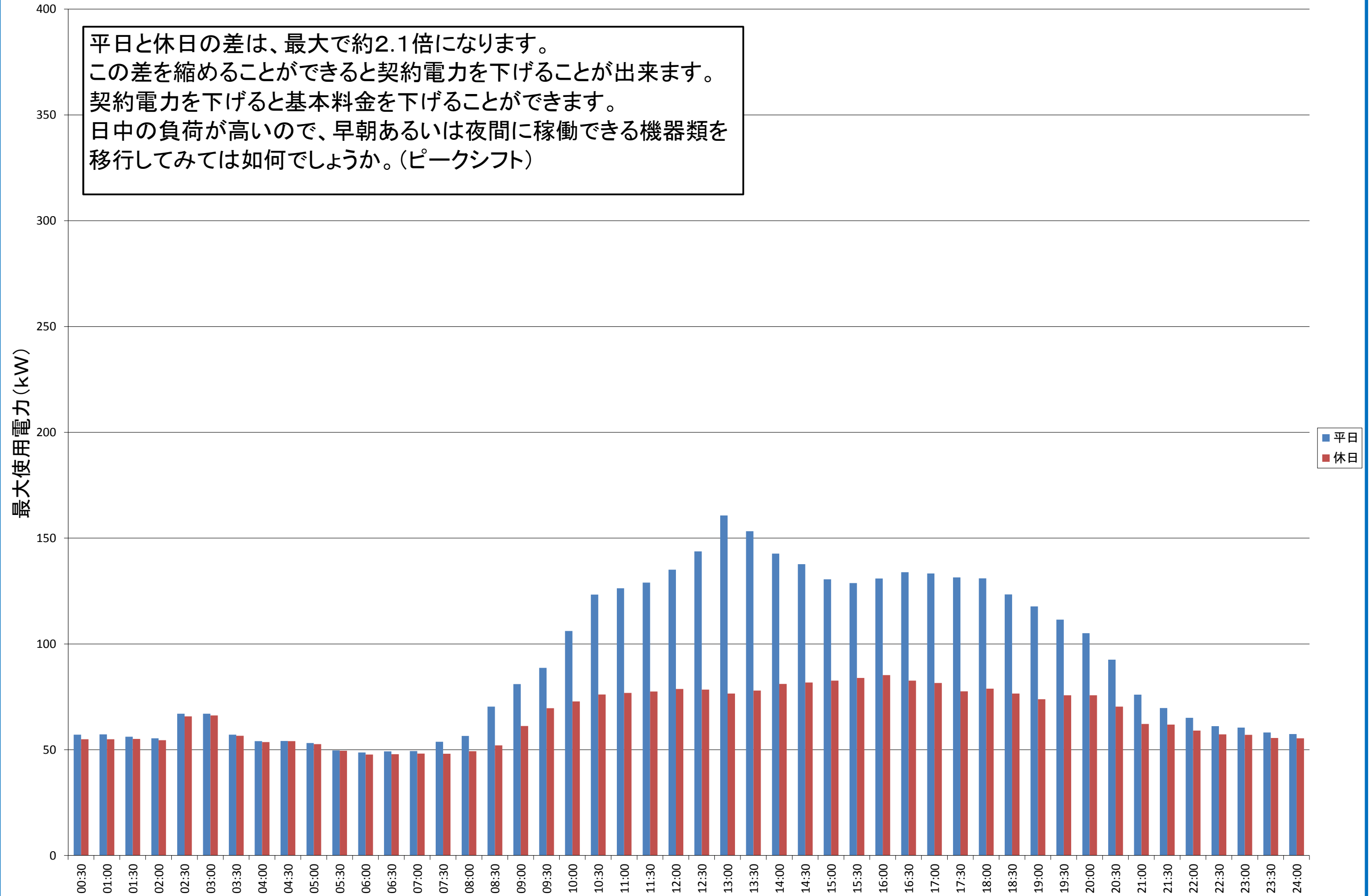
本荘南キャンパス 6月の時間帯別最大使用電力平均値
