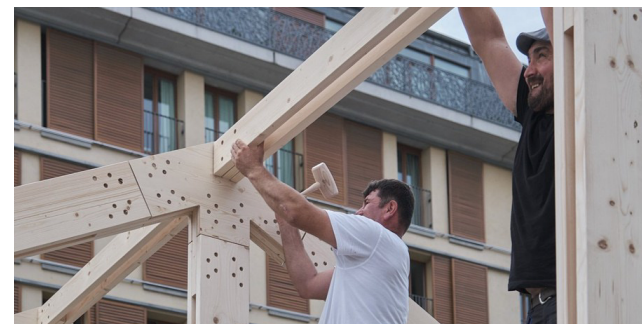
ドイツのフランクフルトで設計した簡易ハウス。接合部に木の「込み栓」を使用
