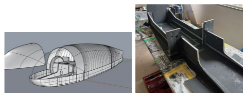
現在制作中の新車両の完成予想図と製作途中の様子です。カーボン製ボディに加えて空気抵抗の少ない流線形の車両にすることで更なる記録の更新を図っています
